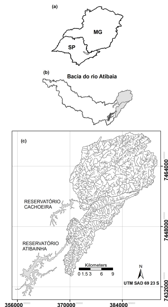
Figura 1. Localização da área de estudos no Estado de São Paulo e Minas Gerais (a), localização das bacias do Cachoeira e Atibainha na bacia do rio Atibaia (b) e as bacias do Cachoeira e Atibainha a montante dos reservatórios (c).
