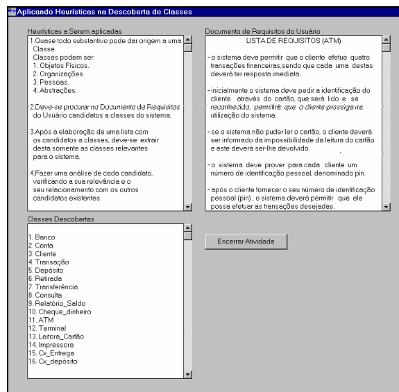
Figura 8. Aplicando heurísticas na descoberta de classes
