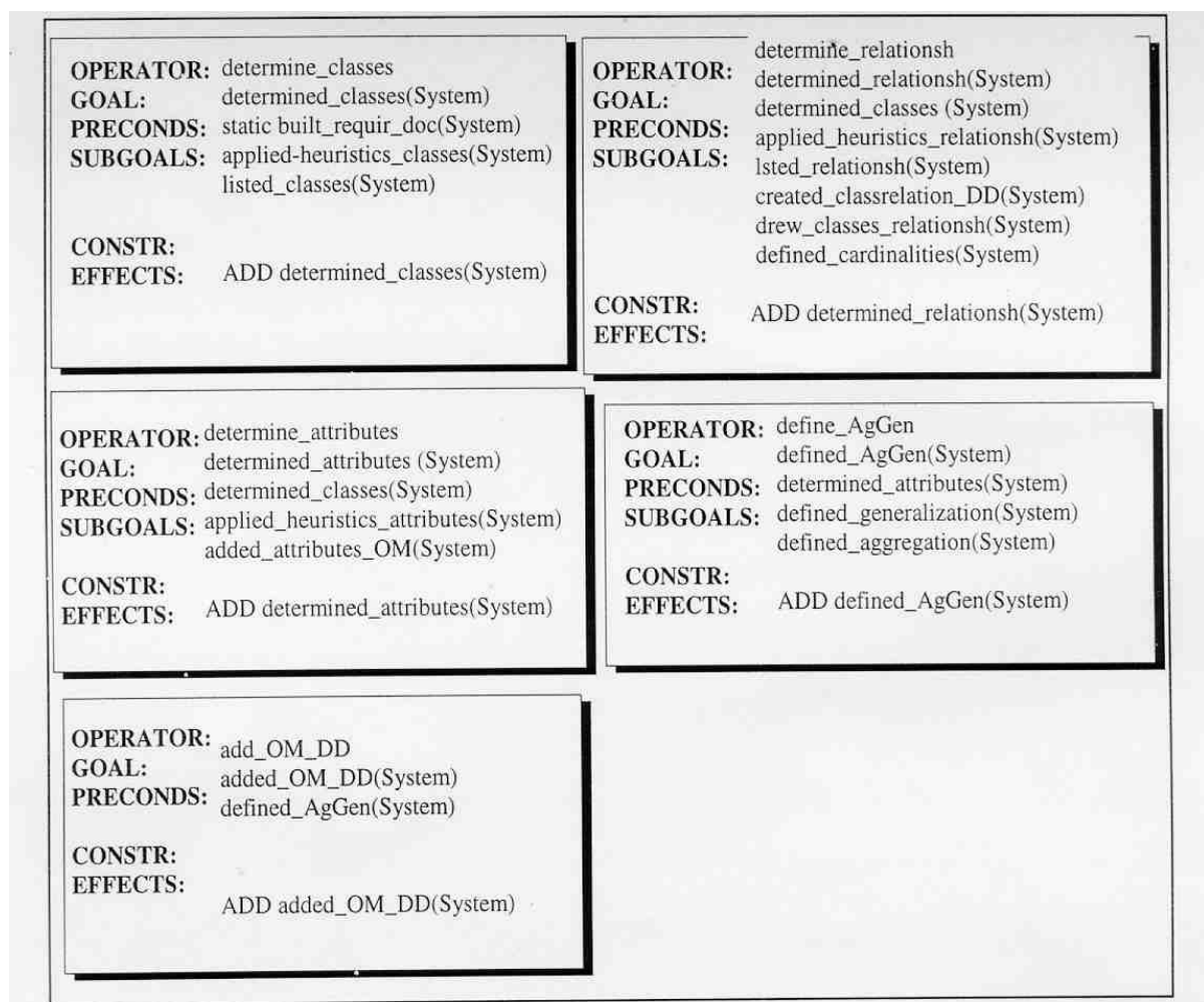
Figura 4. Segundo nível de operadores para create_obj_mod
