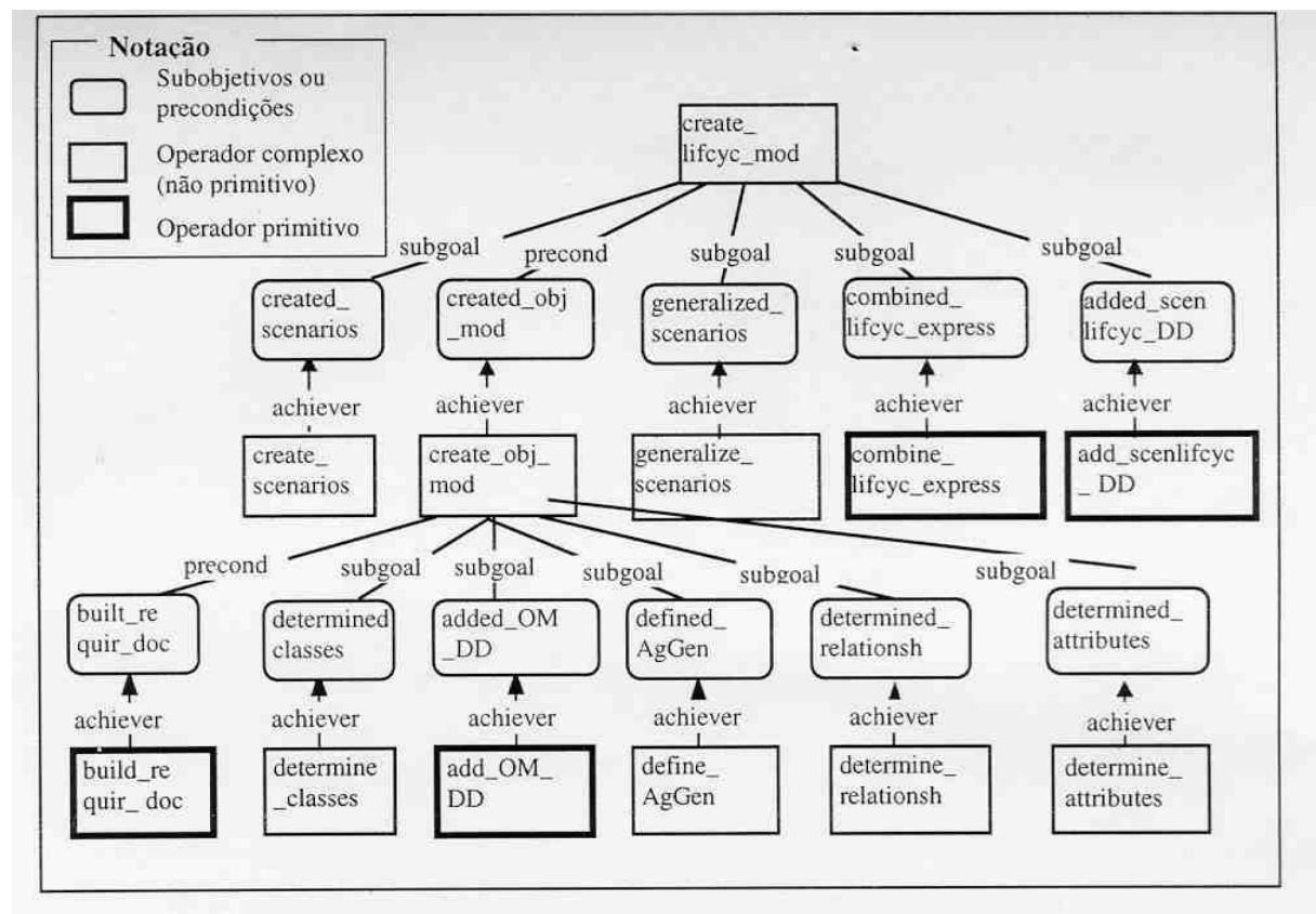
Figura 5. Uma visão de operador do método Fusion
