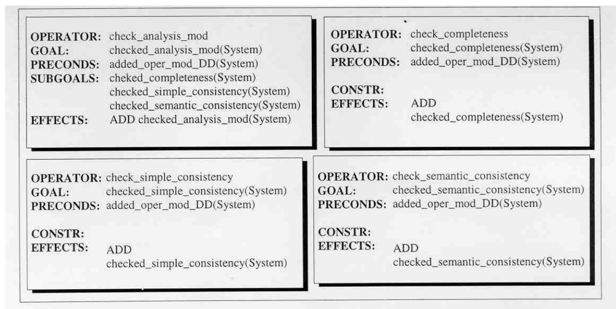
Figura 9. Operadores das verificações dos modelos da fase de análise
