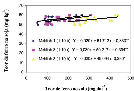
Figura 2. Correlações entre teores de ferro na soja e ferro no solo, extraídos pelo Mehlich 1(1:10 b) com filtragem após decantação, Mehlich 3 (1:10 a), com filtragem imediata e Mehlich 3 (1:10 b), com filtragem após decantação.
