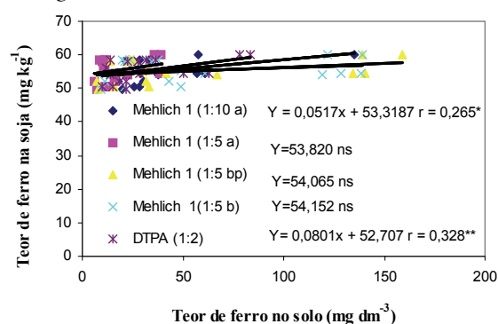
Figura 1. Correlações entre teores de ferro na soja e ferro no solo, extraídos pelo Mehlich 1 (1:10 a), com filtragem imediata, Mehlich 1 (1:5 a), com filtragem imediata, Mehlich 1 (1:5 bp), com pipetagem após decantação, Mehlich 1 (1:5 b), com filtragem após decantação e DTPA (1:2) com filtragem imediata.
