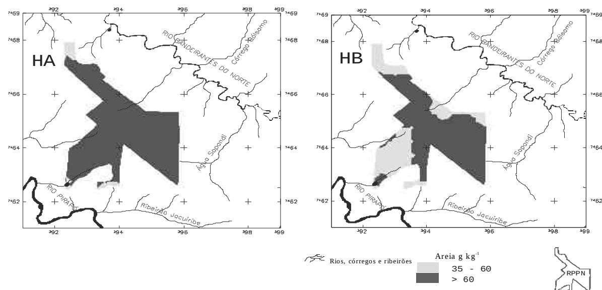
Figura 2. Atributo areia representado nos horizontes A e B, de acordo com a classificação gerada pela análise do modelo numérico do terreno.
