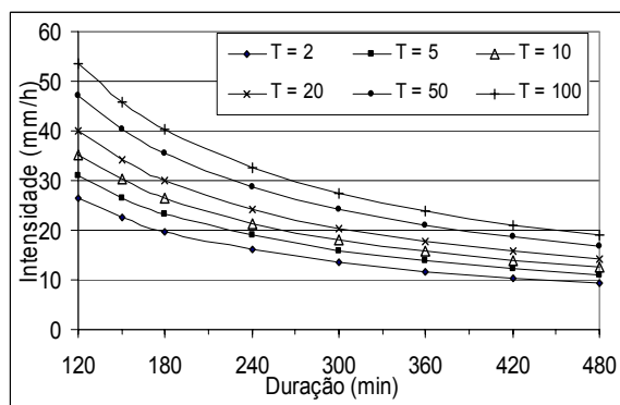
Figura 2. Relação IDF de Chapecó, Estado de Santa Catarina, para chuvas de duração entre 120 e 480 minutos.
