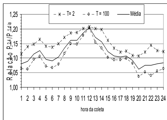
Figura 4. Variação diária da relação entre a precipitação máxima em 24 horas e a precipitação máxima de um dia.
