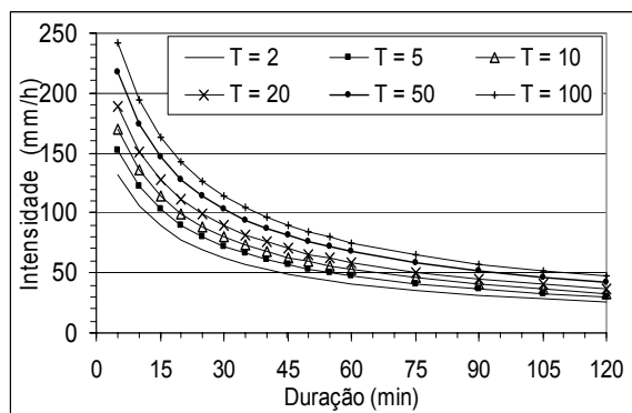
Figura 1. Relação IDF de Chapecó, Estado de Santa Catarina, para chuvas de duração inferior a 120 minutos.
