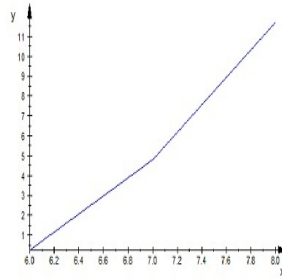
Figura 4: Valores del BR(K_{1,k}, Z_n) para k = 3 fijo y 6 \leq n \leq 8
