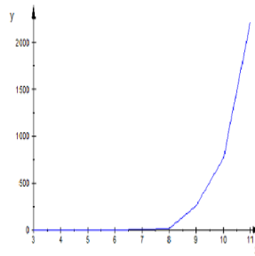
Figura 1: Valores del BR(K_{1,k}, Z_n) para k = 3 fijo y 3 \leq n \leq 11
