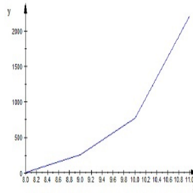
Figura 3: Valores del BR(K_{1,k}, Z_n) para k = 3 fijo y 8 \leq n \leq 11
