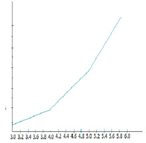
Figura 2: Valores del BR(K_{1,k}, Z_n) para k = 3 fijo y 3 \leq n \leq 6
